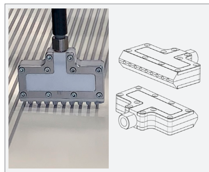
Application unit 2c 100mm (M15x1.5) Gießleiste 2K 100mm (M15x1,5)
