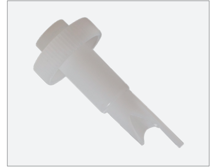
Joint applicator for triangular bead Fugenapplikator für Dreiecksraupe
